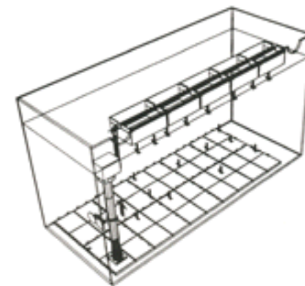
Aquario AUSTRO con cubetas C-1 y filtro de fondo
